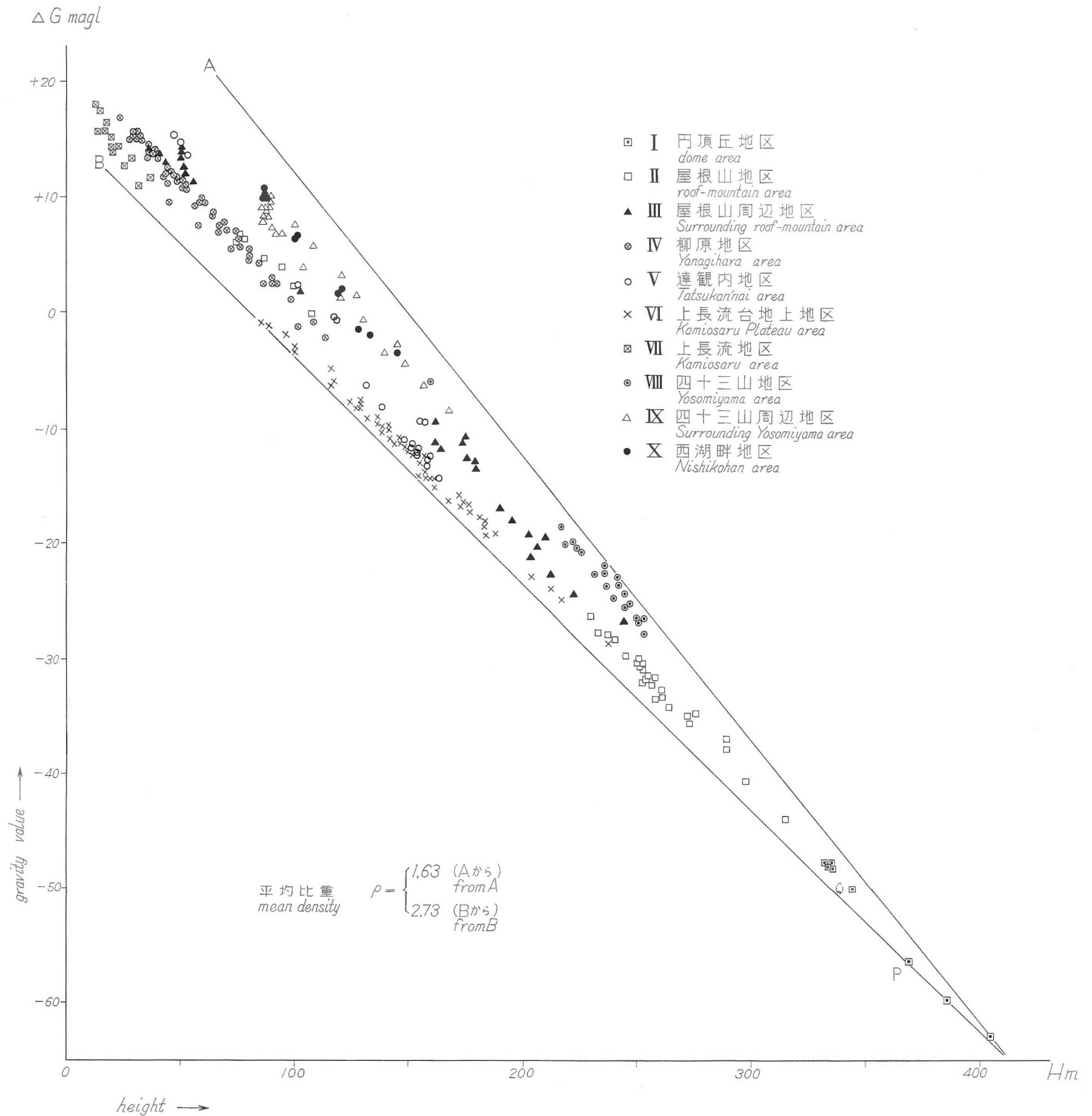
第6図 重力値と高さとの関係 Relation between Gravity Values and Heights
