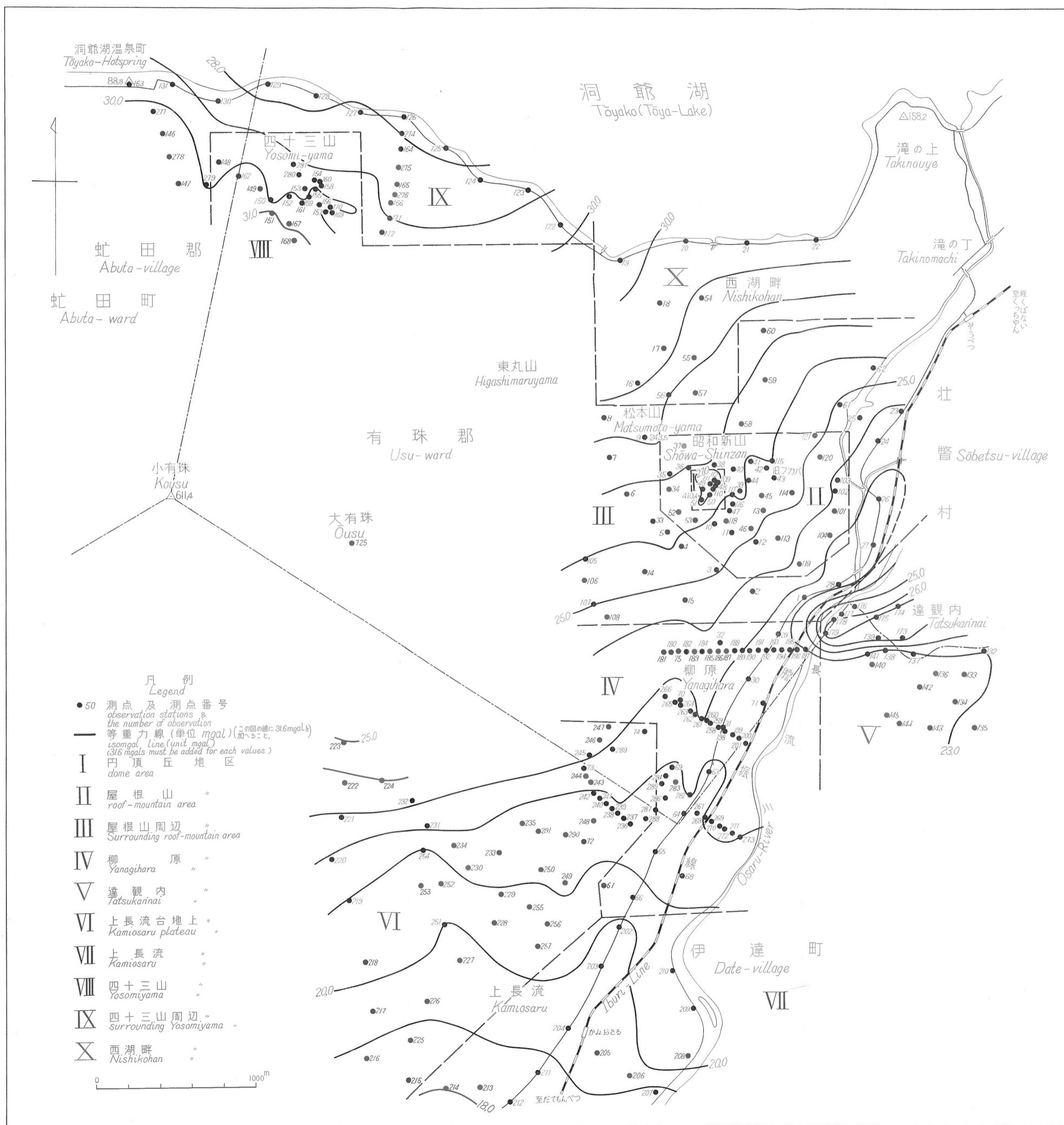
第5図 ブーゲー異常図 Bouguer Anomalies at and near Shōwa-Shinzan
