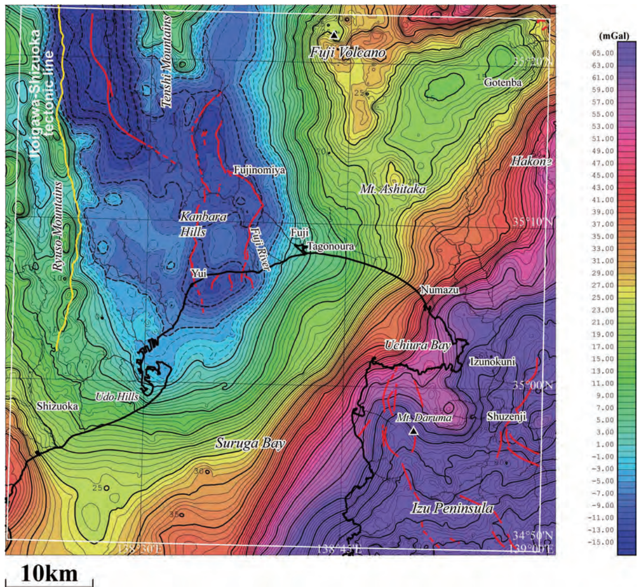
第2図 駿河湾北部沿岸域のブーゲー異常図。仮定密度は 2.3\text{g/cm}^3 。コンター間隔は 1\text{ mGal} 。 実線及び破線のコンターは各々正值と負値を示す。赤の実線：活断層分布（尾崎ほか，2016a）。 Fig.2 Bouguer anomalies in the northern coastal zone of Suruga Bay. Assumed density is 2.3\text{g/cm}^3 . Contour interval is 1\text{ mGal} . Solid and broken lines indicate positive and negative values, respectively. Red solid lines denote active faults after Ozaki et al. (2016a).
