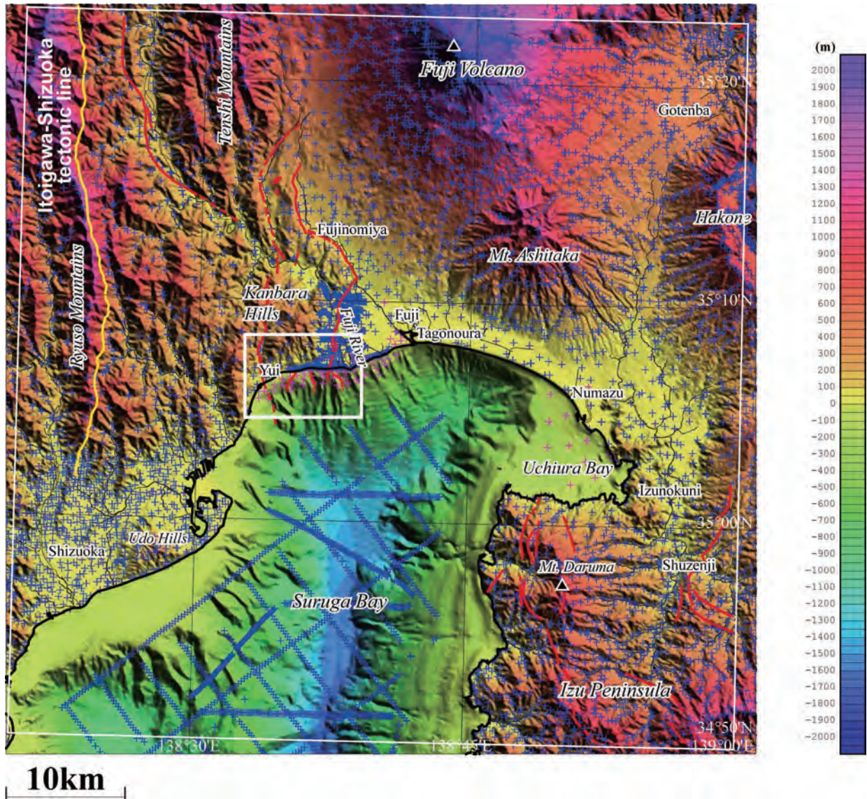
第 1 図 測定点分布図。背景の陰影図は地形。50m メッシュ DEM（国土地理院，1997）と海底地形デジタルデータ（日本海洋データセンター，2012）を使用。 青の十字：既存の重力測点。ピンクの十字：海底重力測点及び新規の陸上測点。 赤の実線：活断層分布（尾崎ほか，2016a）。白の実線で示された矩形は詳細な検討範囲（第 5 図）を示す。 Fig.1 Distribution of gravity stations. Shaded terrain relief is superimposed. The 50m mesh DEM (GSI, 1997) and Bathymetry-Topography Digital Data (JODC, 2012) were used. Blue crosses: Pre-existing gravity stations. Pink crosses: Ocean bottom gravity stations and newly observed land gravity stations. Red solid lines denote active faults after Ozaki et al. (2016a). The rectangle bounded by white solid lines indicates the detailed study area (Fig. 5).
