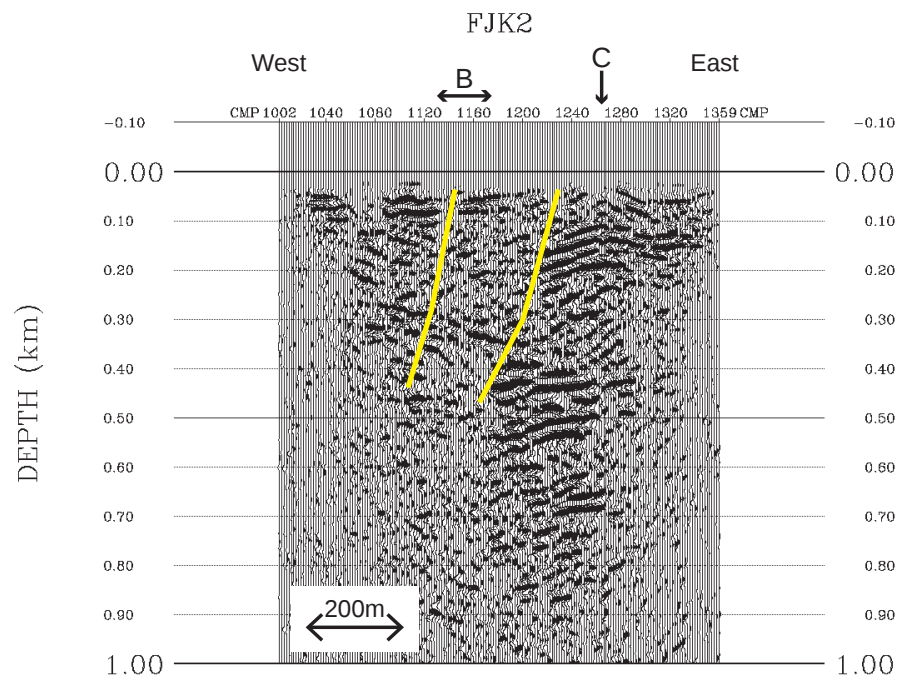
第7図 FJK2 のマイグレーション深度断面. 黄色の曲線は成層構造のずれを示す. B と C はそれぞれ蒲原地震山と中田・今泉編 (2002) による入山瀬断層の位置を示す. Fig. 7 Migrated depth profile of FJK2. Yellow curves indicate gaps of stratification. B and C show locations of Kambara-Jishin-Yama and the Iriyamase Fault by Nakata and Imaizumi (2002), respectively.
