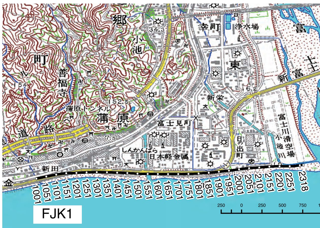
第2図 FJK1 の CMP 位置図。基図に国土地理院発行の数値地図 50,000（地図画像）を使用。
