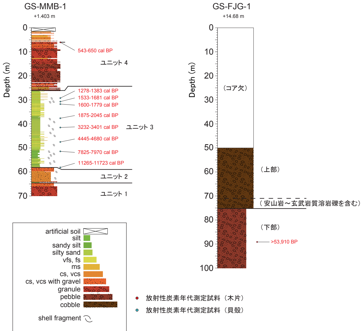
第4図 GS-MMB-1 と GS-FJG-1 の地質柱状図.
