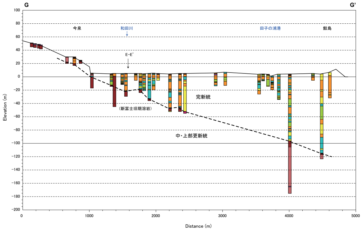
第 13 図 富士川河口部の地質断面 (G-G')。凡例は第 11 図と同じ。断面図の位置は第 3 図参照。
