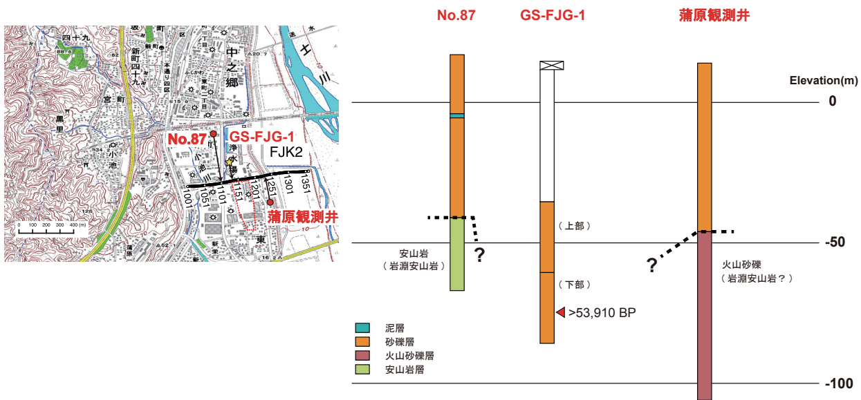
第 14 図 FJK2 測線に沿った GS-FJG-1 近傍の断面。地図は伊藤・山口 (2016) に加筆。
