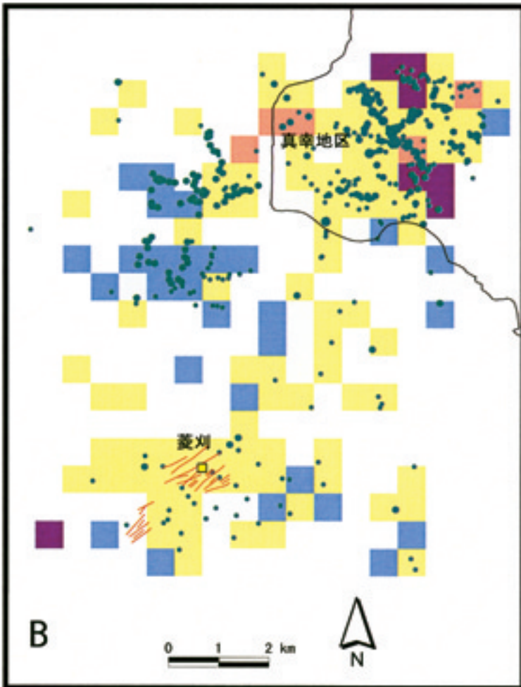
串木野鉱床地区 (A) と菱刈鉱床地区 (B) の変質と岩石の金含有量の比較図。 広域調査データベースについての説明は、本文63頁囲み記事を参照されたい。
