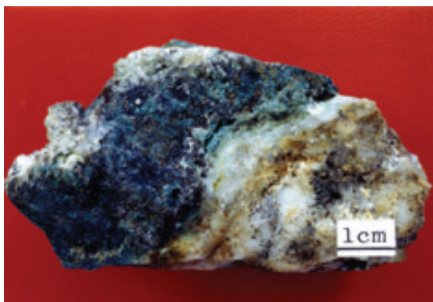
2. 芹ヶ野金山(後の串木野金山)向田ひ(?)の金銀鉱石. 高銀倍率と推定される. 白色部は石英と氷長石. エレクトラム(金銀合金鉱物)や, 銀, 銅, 鉄などの金属の硫化鉱物が多く含まれている銀黒部の表面に緑色の二次銅鉱物. 明治後期に採取された. 尚古集成館の標本.
