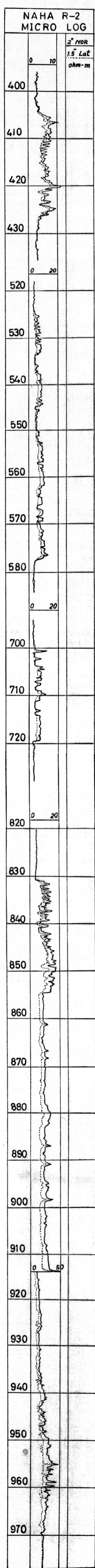
第16図 電気検層図 (c, マイクロ) Electric log of Naha R-2 Test Well (c)
