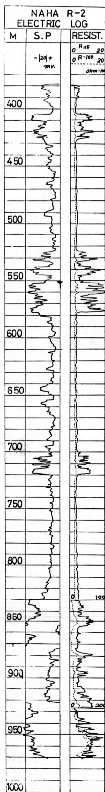
第15図 電気検層図 (b, 深部) Electric log of Naha R-2 Test Well (b)
