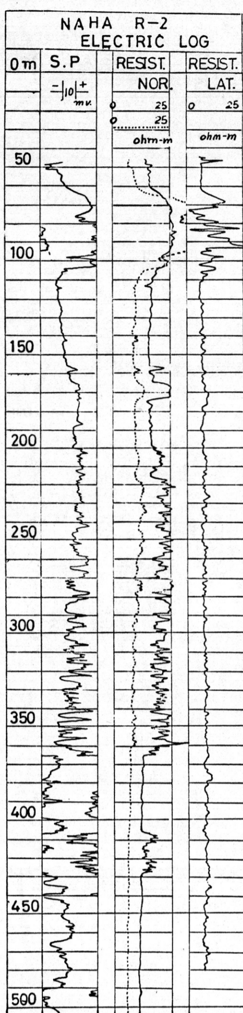
第14図 電気検層図 (a, 浅部) Electric log of Naha R-2 Test Well (a)
