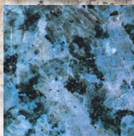
花崗岩：上から ラバキヒ花崗岩、赤色花崗岩、青色閃長岩
