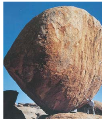
ナミビアの巨大な花崗岩ボール 永田助親氏撮影
